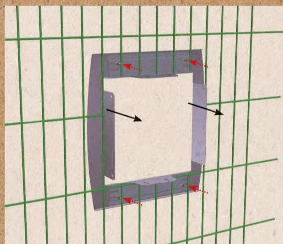
2 - Placer les vis aux 4 extrémités du cadre avant et positionner le cadre sur la clôture.
