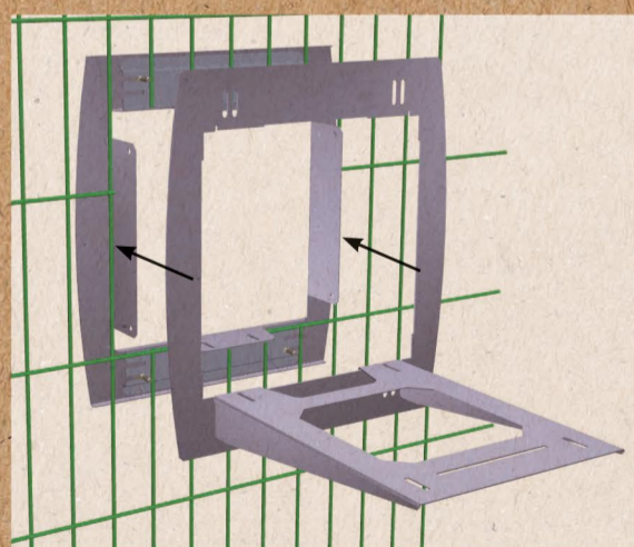
4 - Puis assembler le tout en alignant les 2 cadres.
