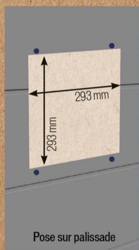
1 - Faire une réservation de 293 x 293 mm à l'aide du gabarit de découpe fourni (marques rouges). Veiller à ce que la réservation se trouve à 1000 mm du sol. Pour les palissades, percer les 4 trous selon les repères (marques bleues).
