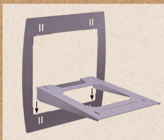
3 - Clipper d'abord le plancher sur le cadre arrière.
