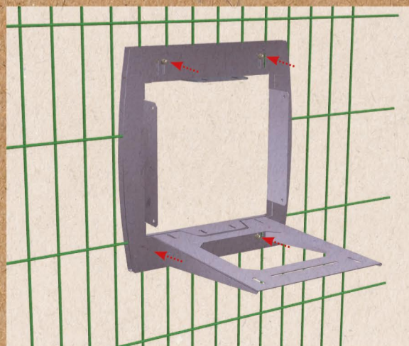
5 - Fixer à l'aide des 4 écrous. Choisir la visserie en fonction de l'épaisseur de la clôture.
