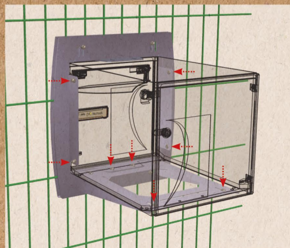
6 - Placer la boîte et ajuster le positionnement. Fixer la boîte sur le support à l'aide des 4 vis, rondelles et écrous. Percer la boîte des deux côtés et fixer à l'aide des 4 vis et écrous borgnes.
