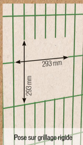
1 - Faire une réservation de 293 x 293 mm à l'aide du gabarit de découpe fourni (marques rouges). Veiller à ce que la réservation se trouve à 1000 mm du sol. Pour les palissades, percer les 4 trous selon les repères (marques bleues).
