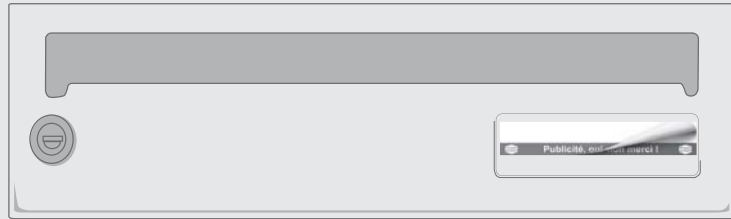
modèle FLat 110 largeur 370 mm - hauteur 110 mm
